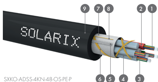
SXKO-ADSS-4KN-48-OS-PE-P
